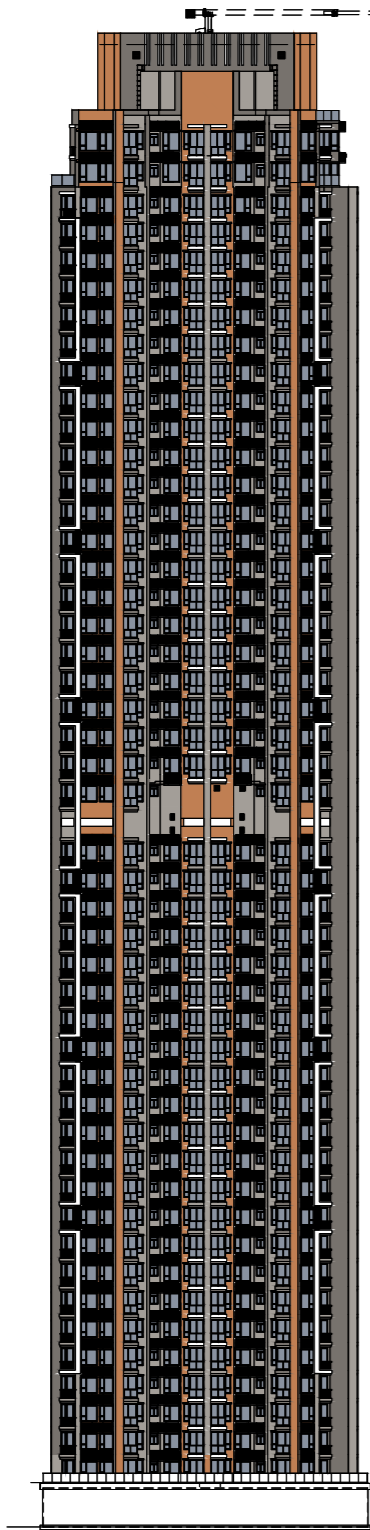
ELEVATION 4 立面圖 4
