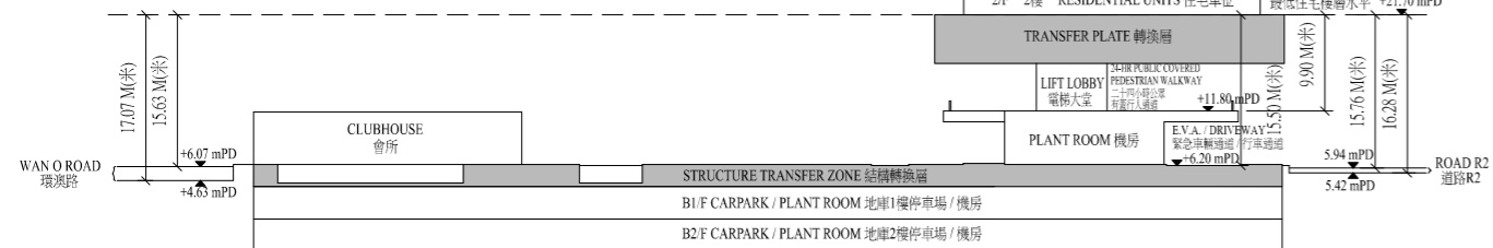
CROSS - SECTION PLAN A 橫截面圖 A
